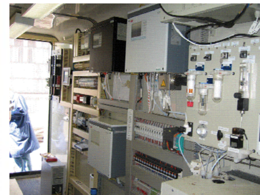
TERMOELEKTRARNA Šoštanj, Šoštanj, Blok 5 AMS: CO, NO, SO 2 , O 2 , TOC
